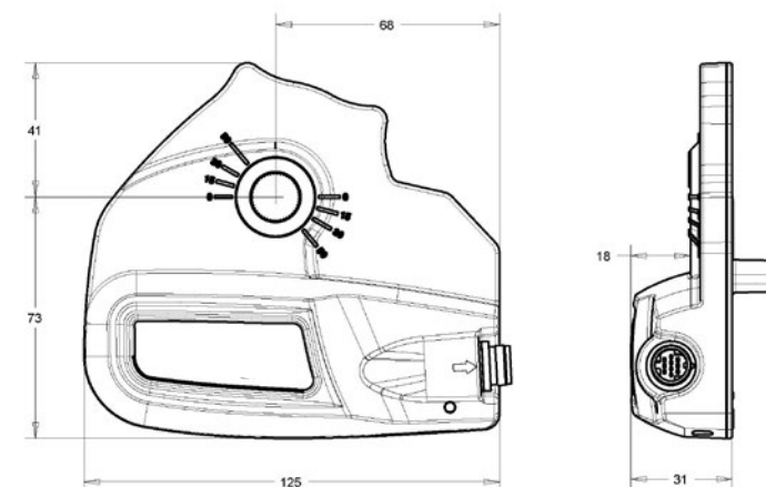
Interfaz del cojinete Harmony
