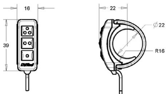
Controlador H3
