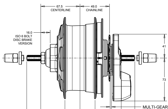
CVP con la interfaz del cojinete Harmony
