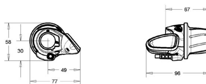
Controlador H8
