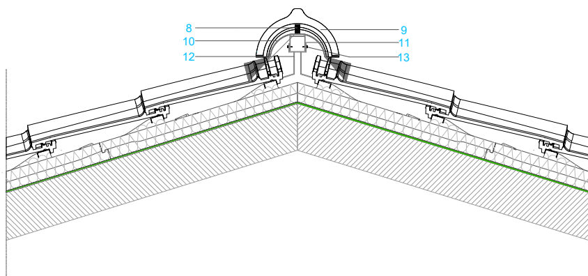
CORTE 1
