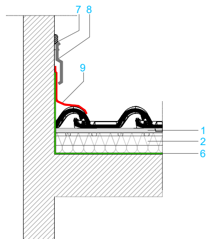
CORTE 2 REIMATE COM PAREDE LATERAL
