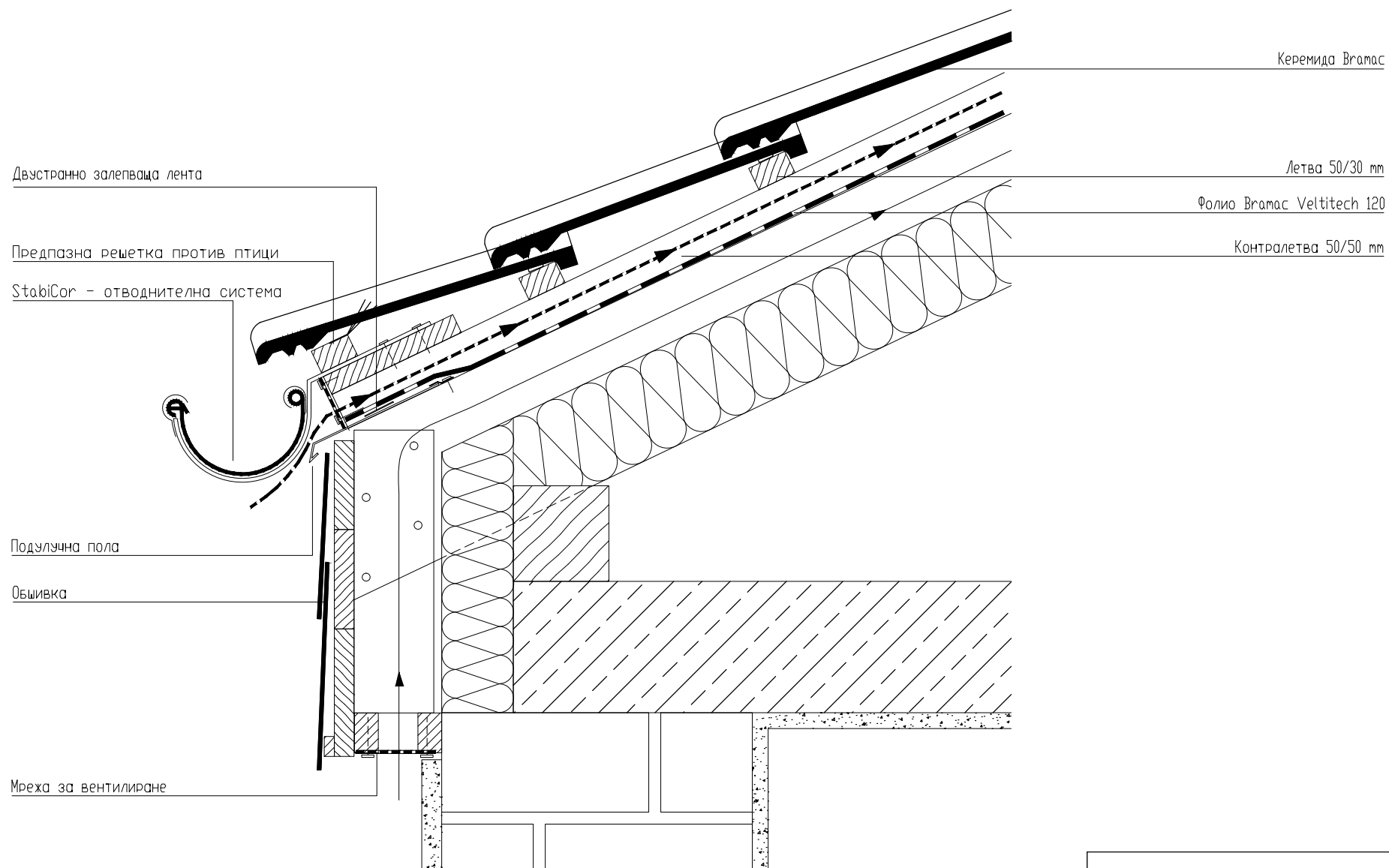
Детайл на стреха завършване на реброто с челна обшивка Брамак Покривни Системи ЕООД Дата: 06/2010 Мащаб: 1 : 5
