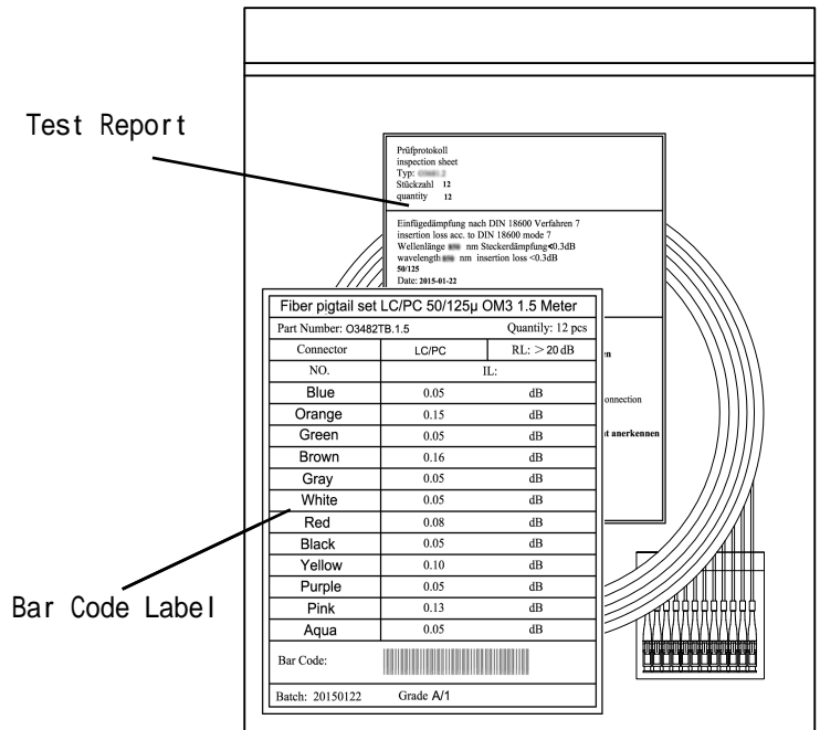
PE Bag(150mm x 140mm)
