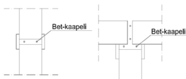
Kuva 12 Betonilämmityskaapelin sijoitus päittäis- ja T-saumoissa
