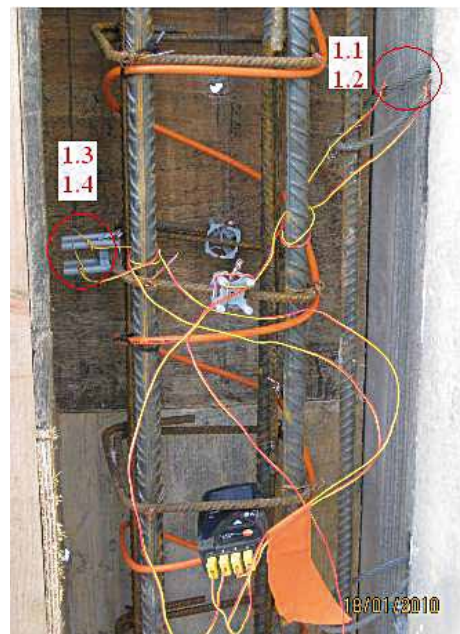
Termolankojen 2.1 – 2.4 sijoitus pilasterissa
