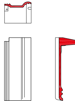
Frankfurter: halve chaperonpan 90°
