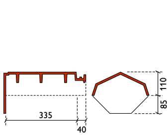
HV beginvorst type K
