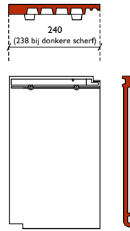
linker eindpan
