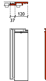
halve pan
