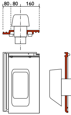
ontluchtingspan met adapter
