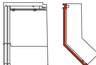
knikgevelpan rechts 140°
