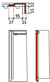
halve gevelpan rechts
