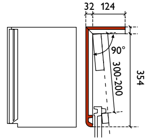
chaperonpan 90° (gezaagd)
