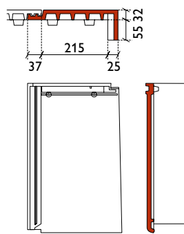
gevelpan rechts
