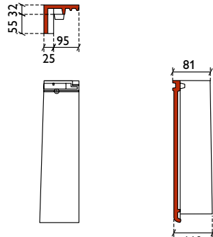
halve gevelpan links
