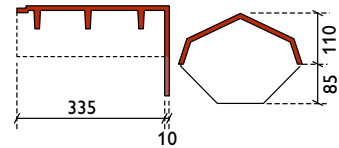
HV eindvorst type K
