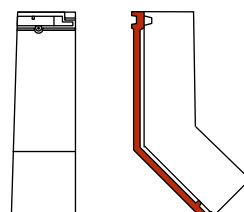
halve knikgevelpan links 140°
