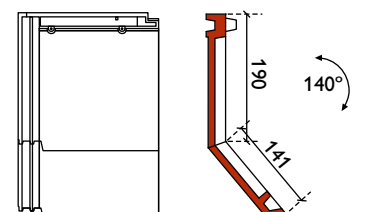
knikpan 140° (gezaagd model)
