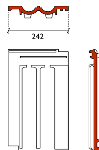
dubbele welpan
