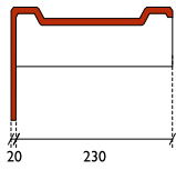
platte eindvorst
