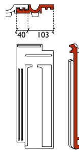
halve pan
