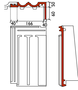
gevelpan rechts
