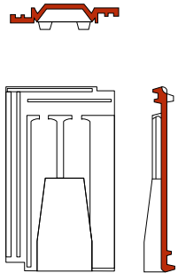
ventilatiepan (ventilatieopening ca. 2.000 mm 2 )
