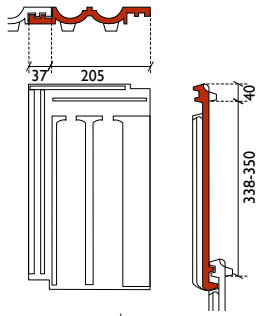
normale pan
