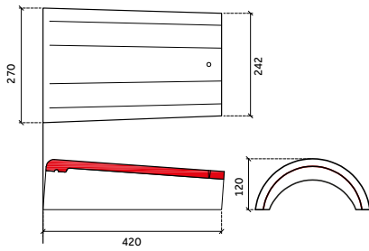
uni-vorst
