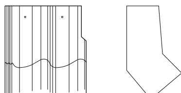
knik gevelpan rechts 140°
