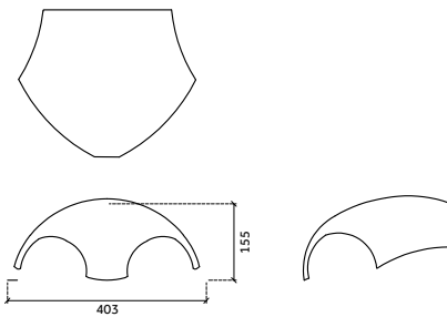
3-zijdig broekstuk
