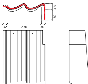
gevelpan rechts
