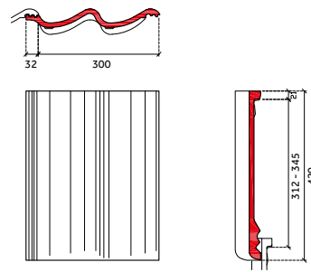
normale pan
