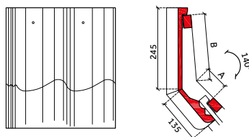
knik pan 140°
