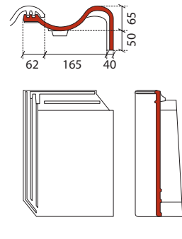
gevelpan rechts
