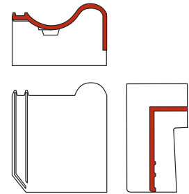
chaperongevelpan rechts 90°
