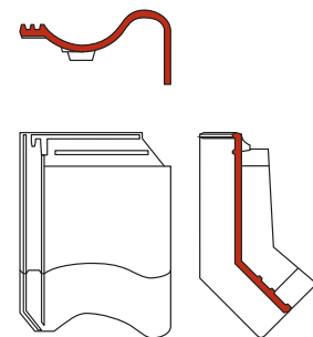
knikgevelpan rechts 140°
