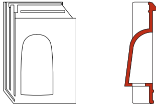
ventilatiepan (ventilatieopening ca. 1.500 mm 2 )
