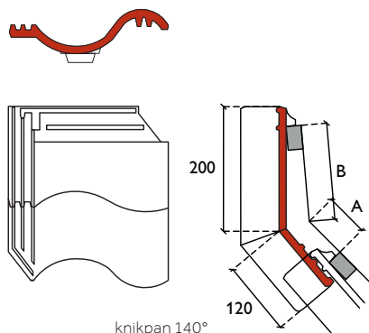
knikpan 140° (gezaagd standaard model)
