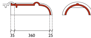
halfronde hoekkeperbeginvorst model Tegelen
