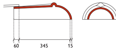
hoekkeperbeginschubvorst model Tegelen
