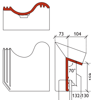
chaperonpan 70° (gezaagd standaard model)
