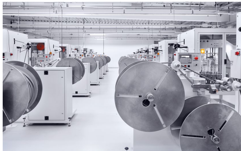
Braiding-Prozess (Ummantelung)
