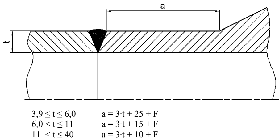
Figur 4-3. Minsta utvändigt fri sträcka från svetsfog
