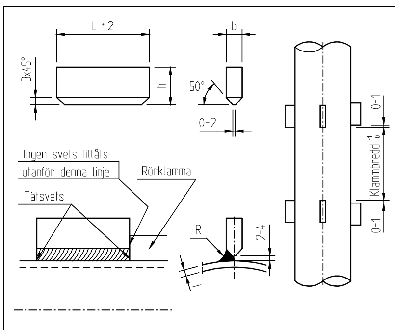
Figur 4-8. Svetsklackar på stålrör
