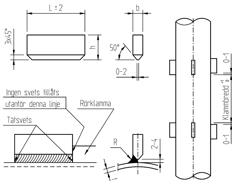
Figur 4-8. Svetsklackar på stålrör
