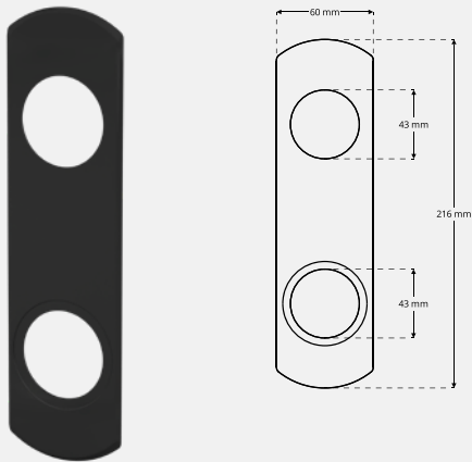
Dækskilt DSP 8774
