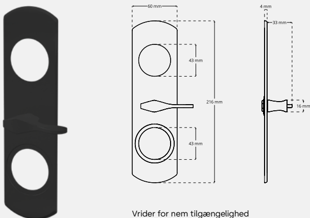
Vrider-dækskilt DSP 8709
