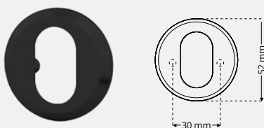
Cylinder roset DR 8320
