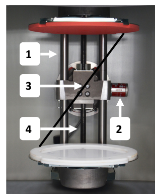
1 Colonnes de guidage 2 Graisseur PERMA 3 Vis sans fin 4 Élastique
