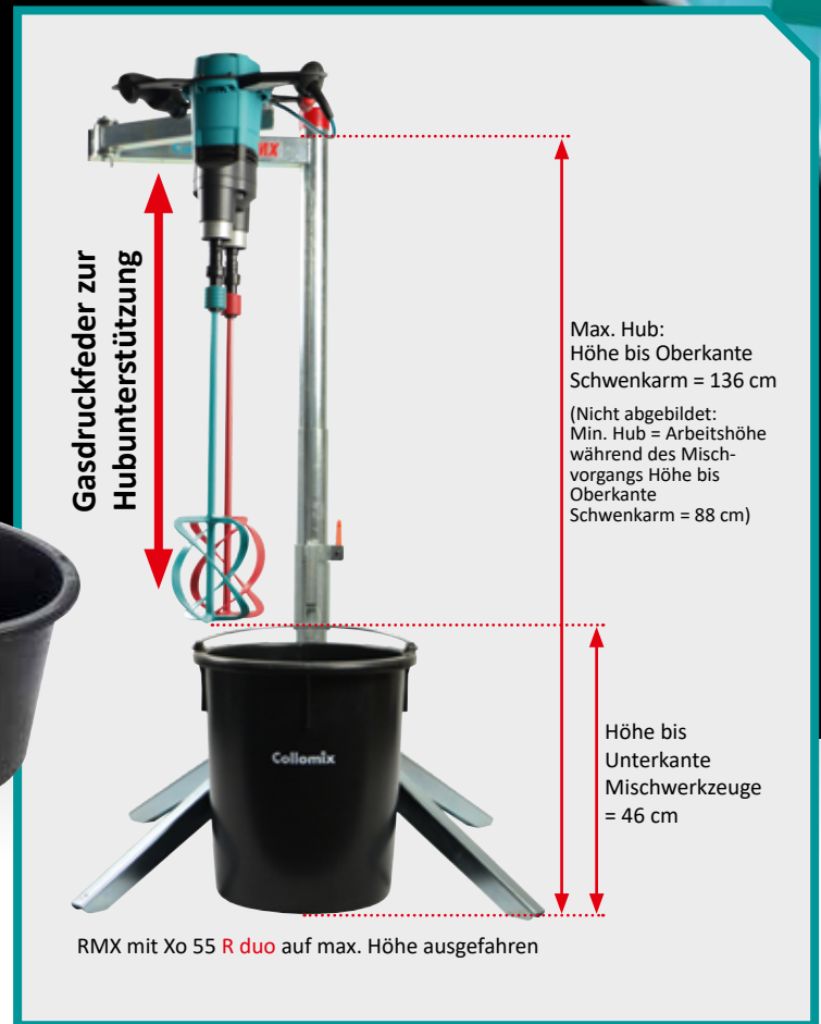
Lieferumfang Rührständer RMX ohne Maschine und Eimer
