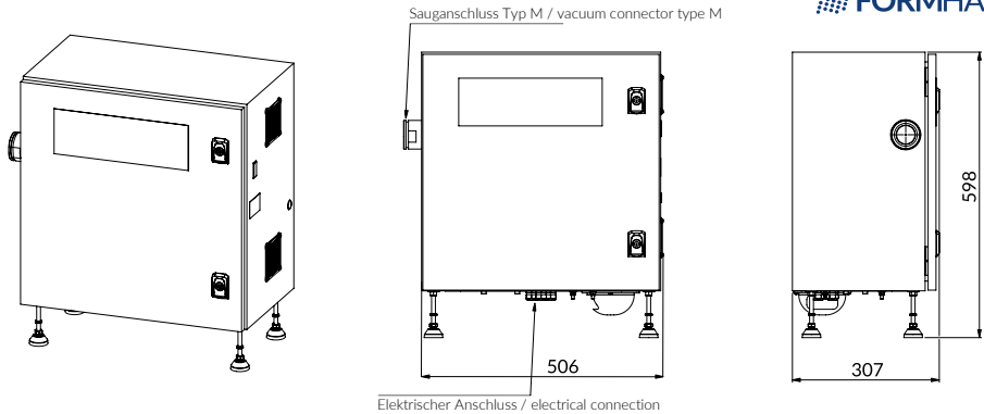
Abbildung: Ansichten des FORMHAND-Saugmoduls S in der Variante S1 Illustration: Views of FORMHAND vacuum module S in variant S1
