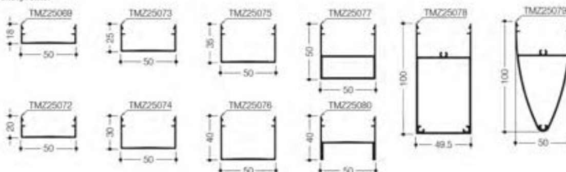
Dekorprofiler
