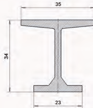
RISKO 134 -profiili.
