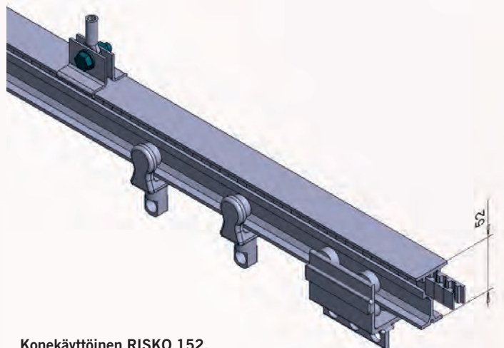
Konekäyttöinen RISKO 152.
