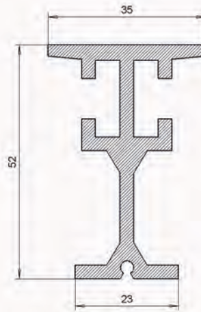
RISKO 152 -profiili.
