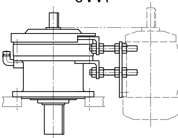
Moottorin asennus sivulle pystyyn
