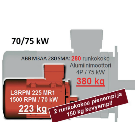
Alumiinirunkoinen oikosulkumoottori ja LSRPM.
