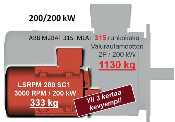
Valurautarunkoinen oikosulkumoottori ja LSRPM.
