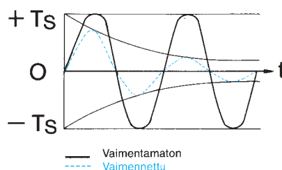
Kuva 4 Vaimennettu ja vaimentamaton vääntömomenttisykäys
