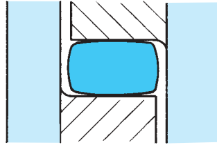
Kuva 2 Kuormitettu polyuretaanihammas
