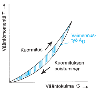
Kuva 3 Progressiivinen vääntöjäykkäyskäyrä
