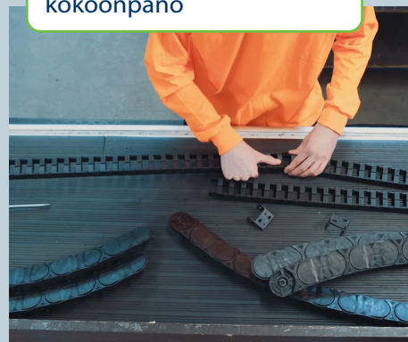
Energiansiirtoketjujen kokoonpano
