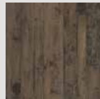
PACAYA MESQUITE Obsidian – PMQ07OBS1
