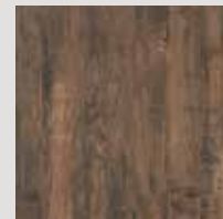
PACAYA MESQUITE Cinder – PMQ07CIN1
