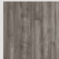
PACAYA MESQUITE Ash – PMQ07ASH1
