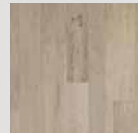
PACAYA MESQUITE Pumice – PMQ07PUM1
