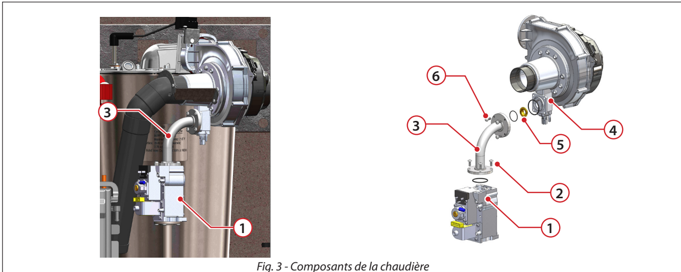
Fig. 3 - Composants de la chaudière
