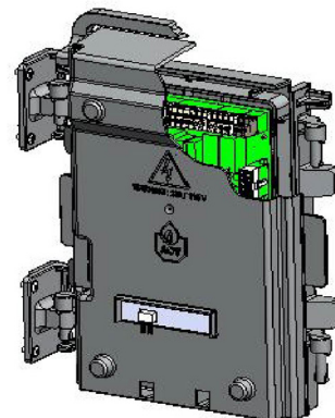
Fig. 8: Prestige Control Module
