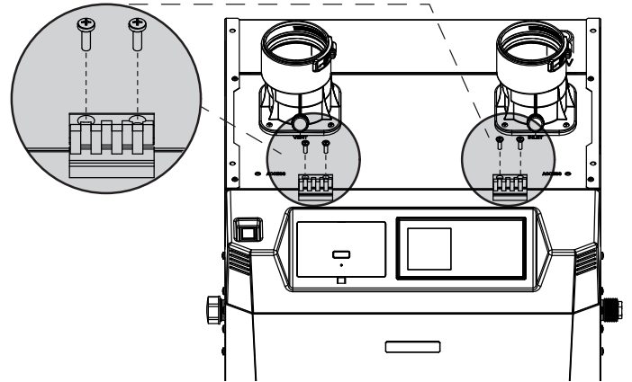
Fig. 10: Hinges
