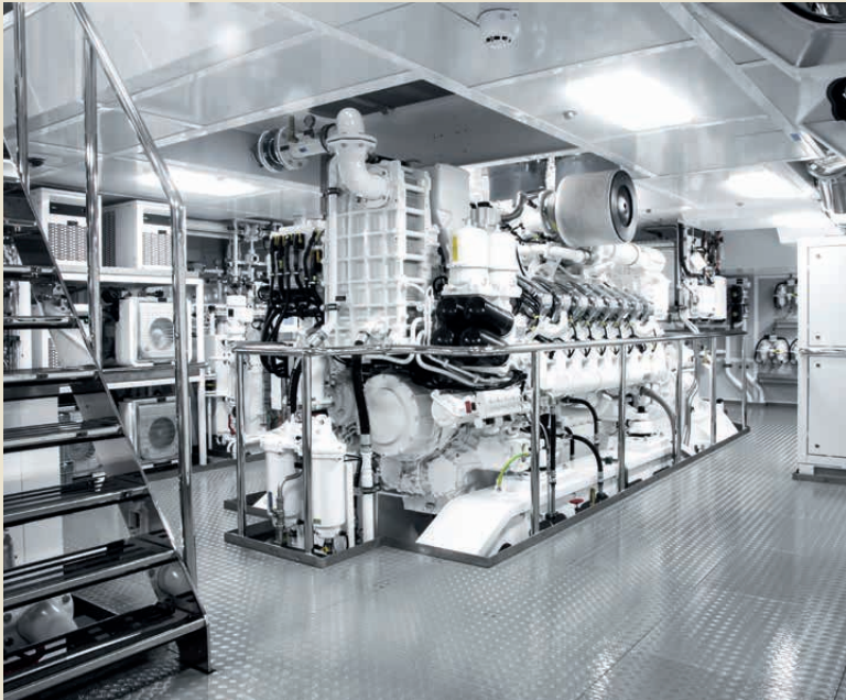
Herzstück: Im Maschinenraum von „Areti“ arbeiten zwei je 2000 kW starke MTU-Motoren. Mit ihnen wird die 85-Meter-Yacht bis zu 17 Knoten schnell.
