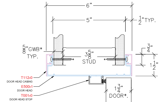
E200 - DOOR HEAD
