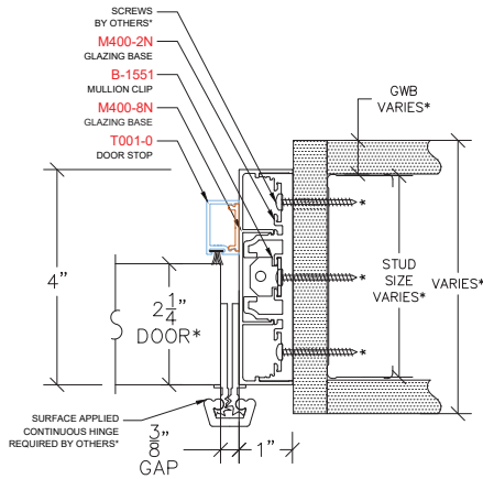
M100 - DOOR JAMB
