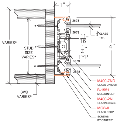
M300 - GLAZING JAMB
