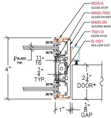
M150 - DOOR JAMB SIDELIGHT
