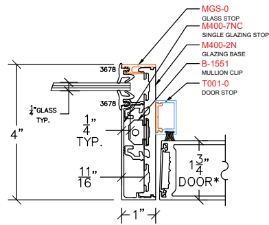
M150 - DOOR JAMB SIDELIGHT
