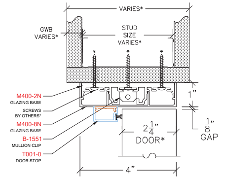
M200 - DOOR HEAD
