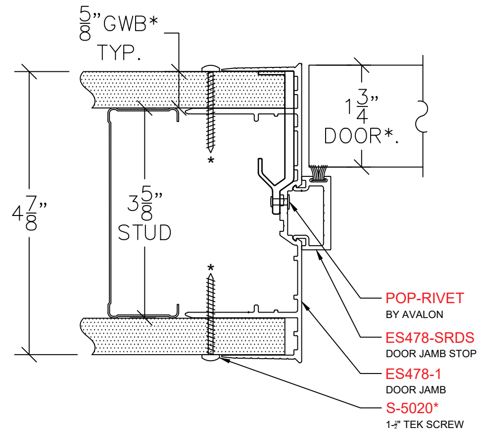
DOOR JAMB CL100
