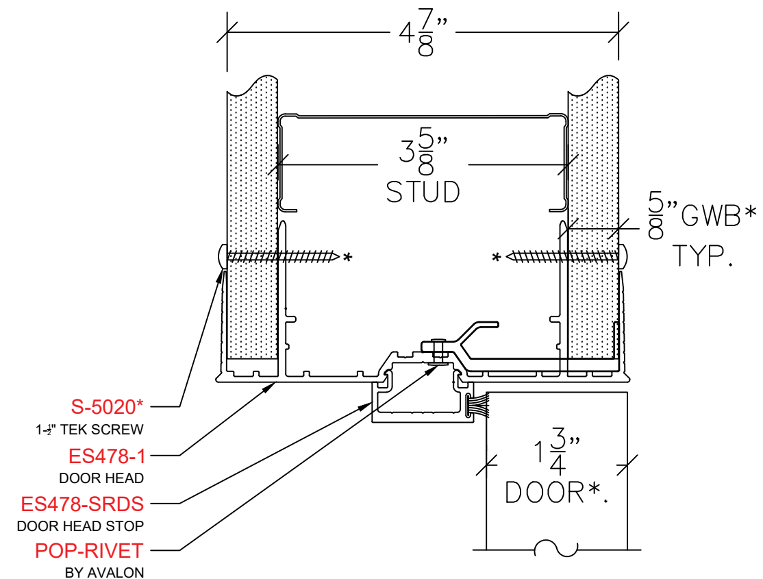
DOOR HEAD CL200
