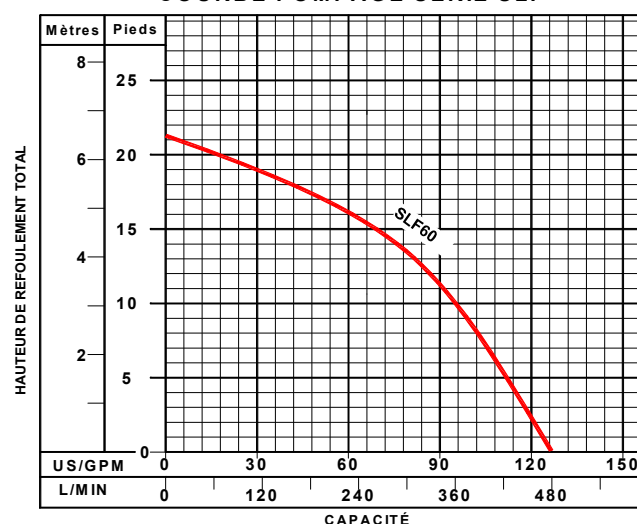
COURBE POMPAGE SÉRIE SLF
