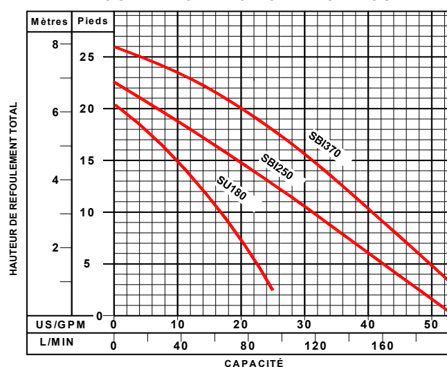
COURBE POMPAGE SÉRIE SBI / SU
