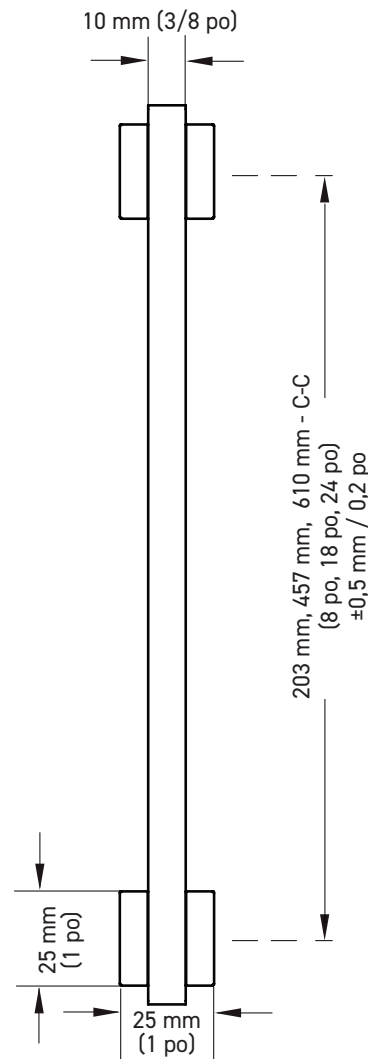
ÉLÉVATION DE FAÇADE
