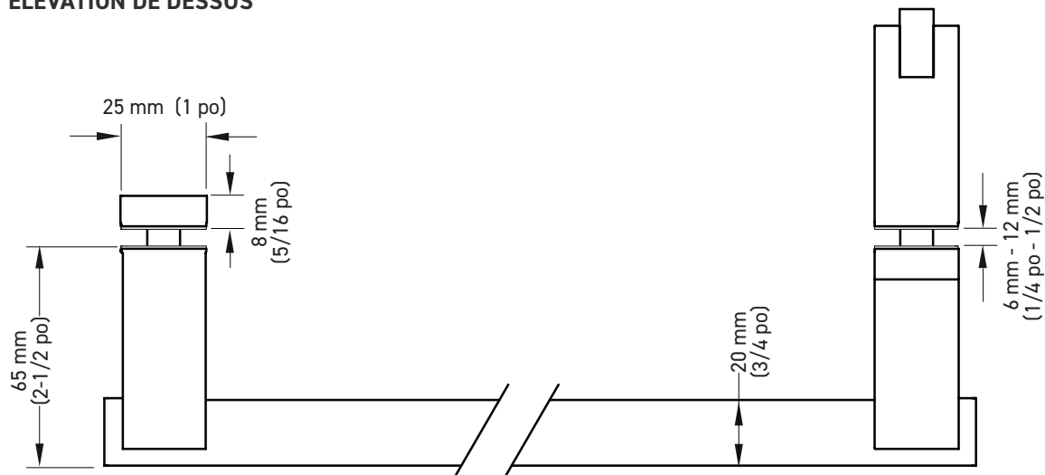
ÉLÉVATION DE DESSUS
