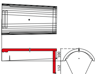
halfronde eindvorst
