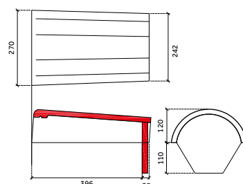
uni-eindvorst
