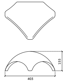
3-zijdig broekstuk
