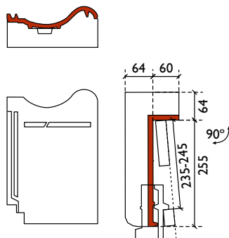
chaperonpan 90° (geperst)
