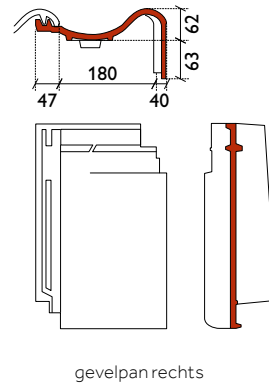
gevelpan rechts
