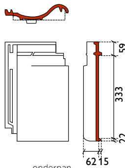
onderpan
