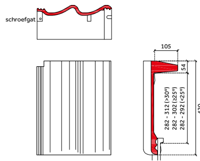
schroefgat
