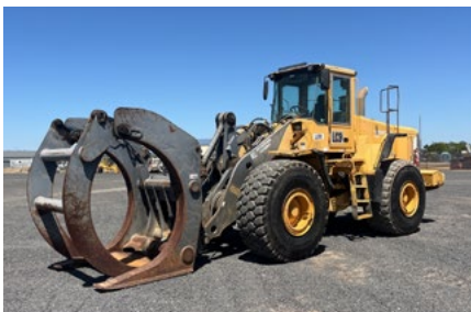
2004 Volvo L150E
