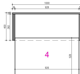
doorsn.
