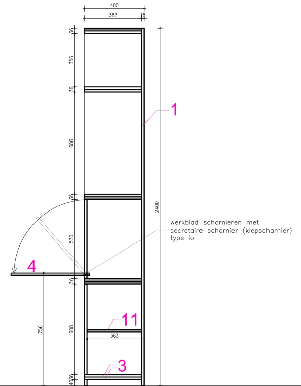
doorsn.
