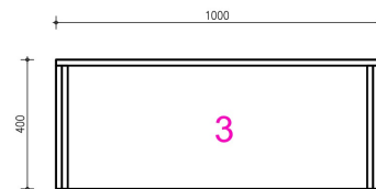
bovenaanzicht
