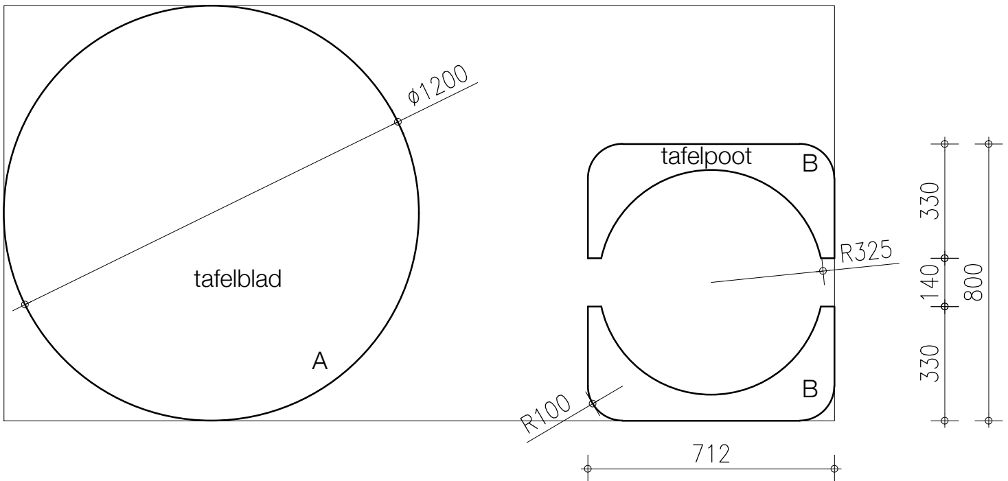
onderdelen tekening
