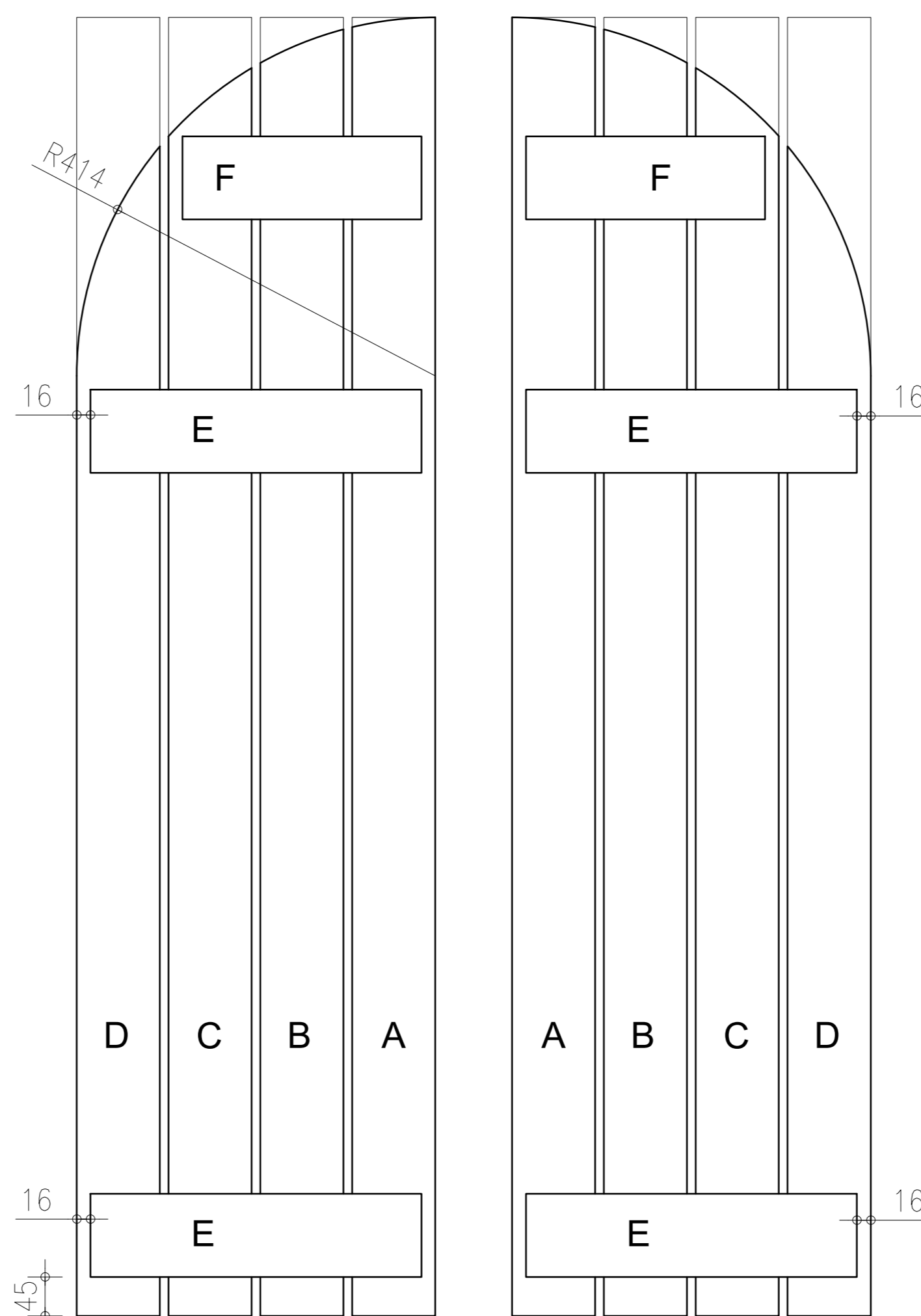
2x deurtje
