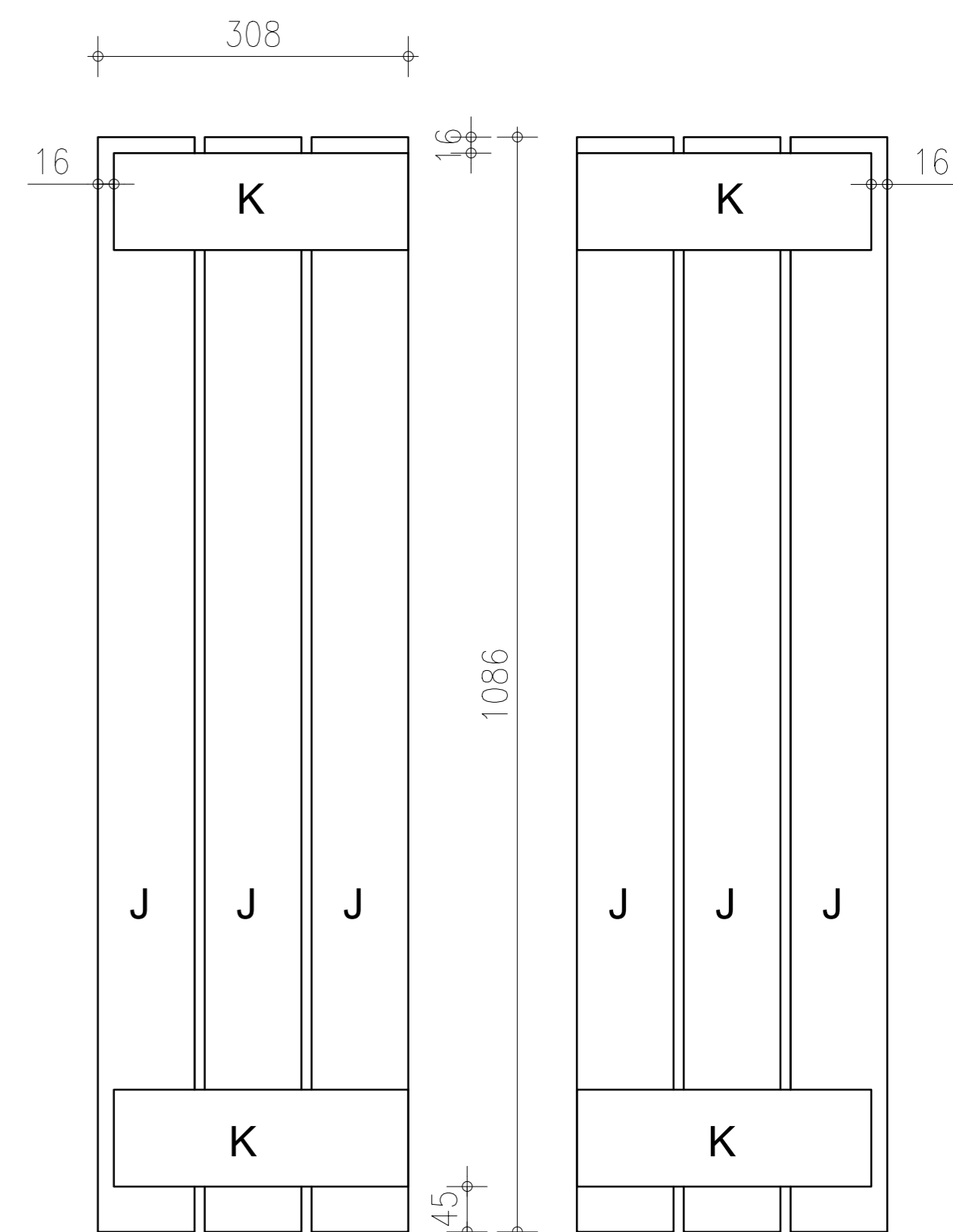
2x zijkant
