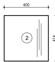
6x zijkanten 400x414x18
