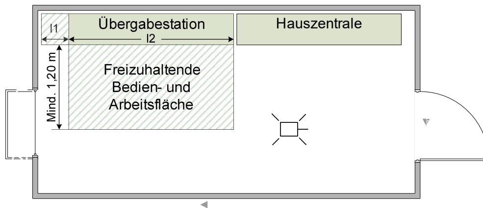
Abbildung 3: Hausanschlussraum
