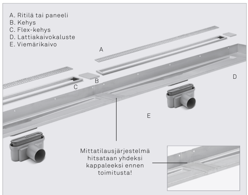
Kuvassa kaksi ClassicLine-kehystä, joiden välissä 120 mm flex-kehys.
