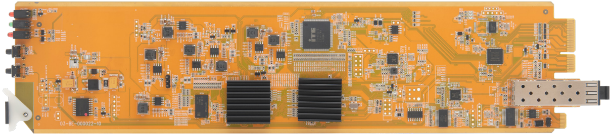
OG-KVM-IP-Tx-UHD-MB
