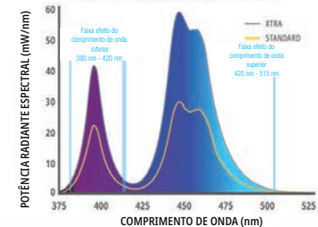
Bandas de comprimentos de onda efetivas para polimerização de compósitos Intervalo de comprimento de onda utilizável: 385 – 515nm
