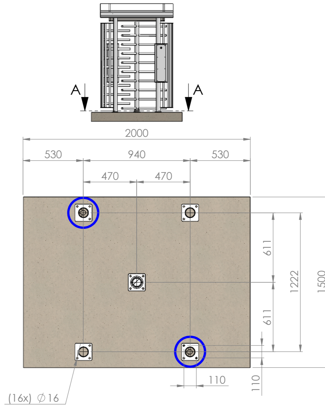
COUPE A-A (VUE DE DESSUS) ECHELLE 1 : 20
