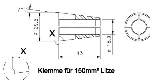
Klemme H6S
