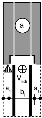
a1 < 50 mm
