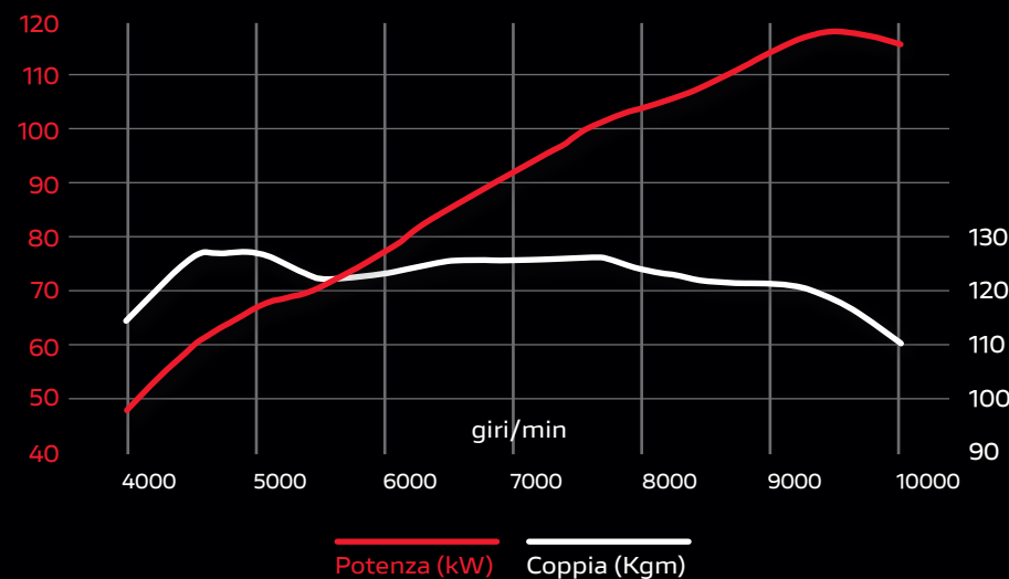
Le curve di coppia e potenza del motore Ducati Testastretta DVT 1262
